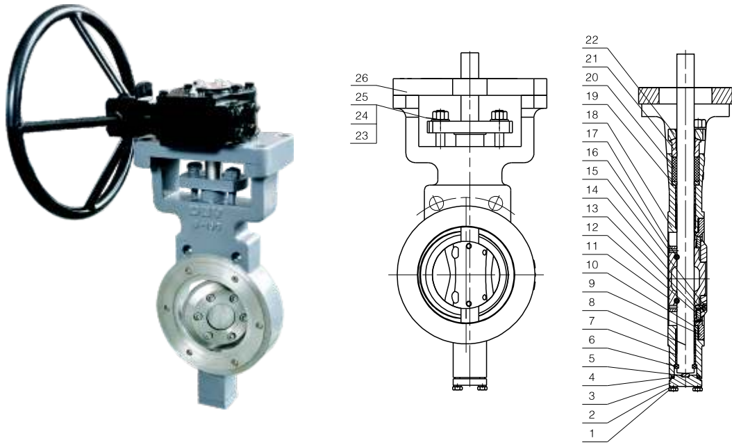
对夹式 Wafer Type
