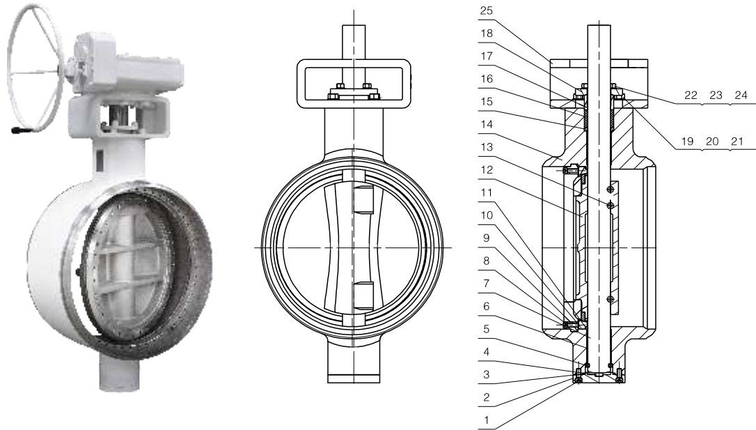
对焊式 Butt weld Type
