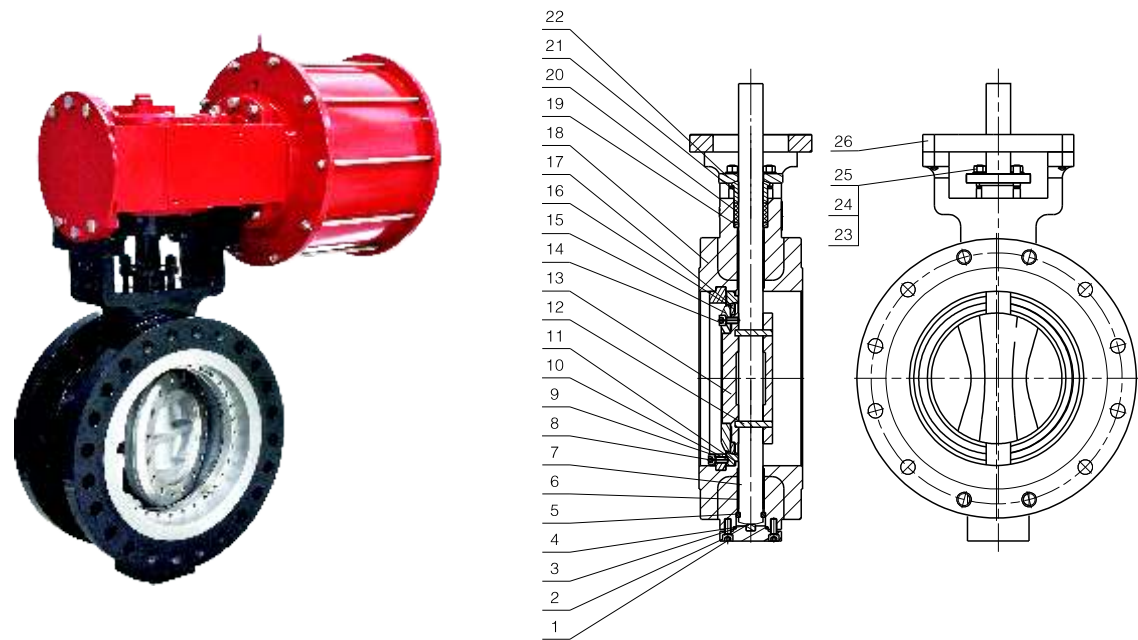
法兰式 Flange Type
